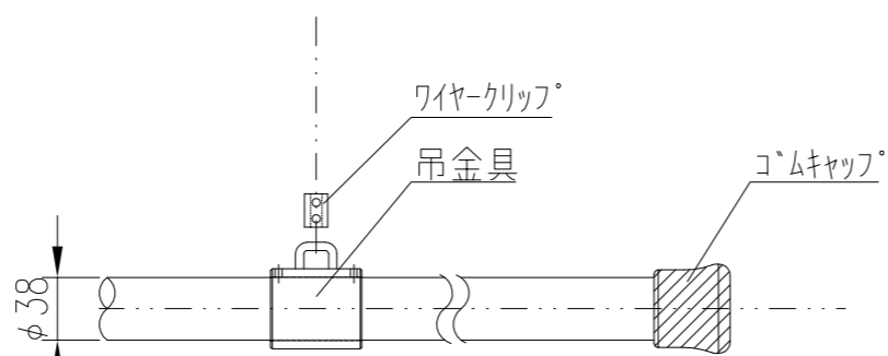
ボタンパイプ詳細図 S=1/5
